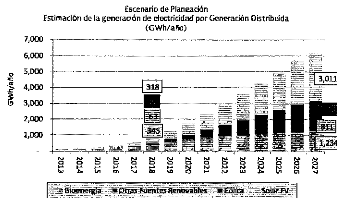
Gráfica 15. Estimación de la generación de electricidad por tecnología para Generación Distribuida (GWh/año)
