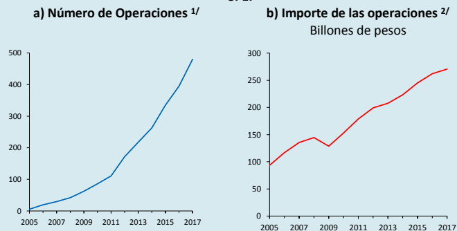
Gráfica 1 SPEI
