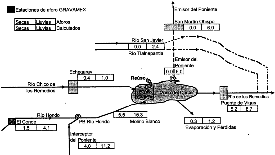
Fig. 9.- Balance de agua con una planta de tratamiento de reúso local de 0.5 m³/s
