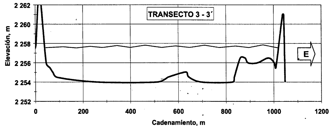
Figs. 6a a 6f.- Perfil de transectos del Vaso El Cristo
